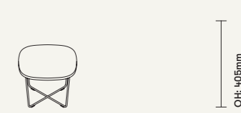
A638-6SS OW: 540mm OD: 540mm
